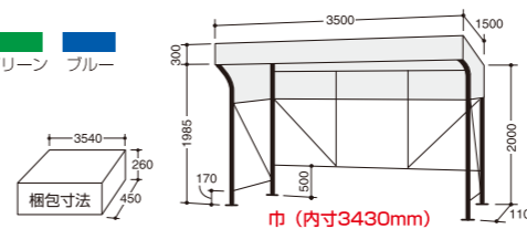
KT-B-35 ¥252,000 (税別) ●テントカラー ■ レッド ■ オレンジ ■ グリーン ■ ブルー
