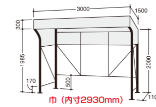
KT-B-30 ¥226,000 (税別) ●テントカラー ■ レッド ■ オレンジ ■ グリーン ■ ブルー
