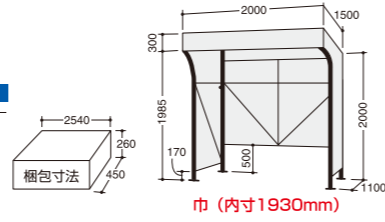
KT-B-20 ¥183,000 (税別) ●テントカラー ■ レッド ■ オレンジ ■ グリーン ■ ブルー
