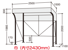
KT-B-25 ¥198,800 (税別) ●テントカラー ■ レッド ■ オレンジ ■ グリーン ■ ブルー
